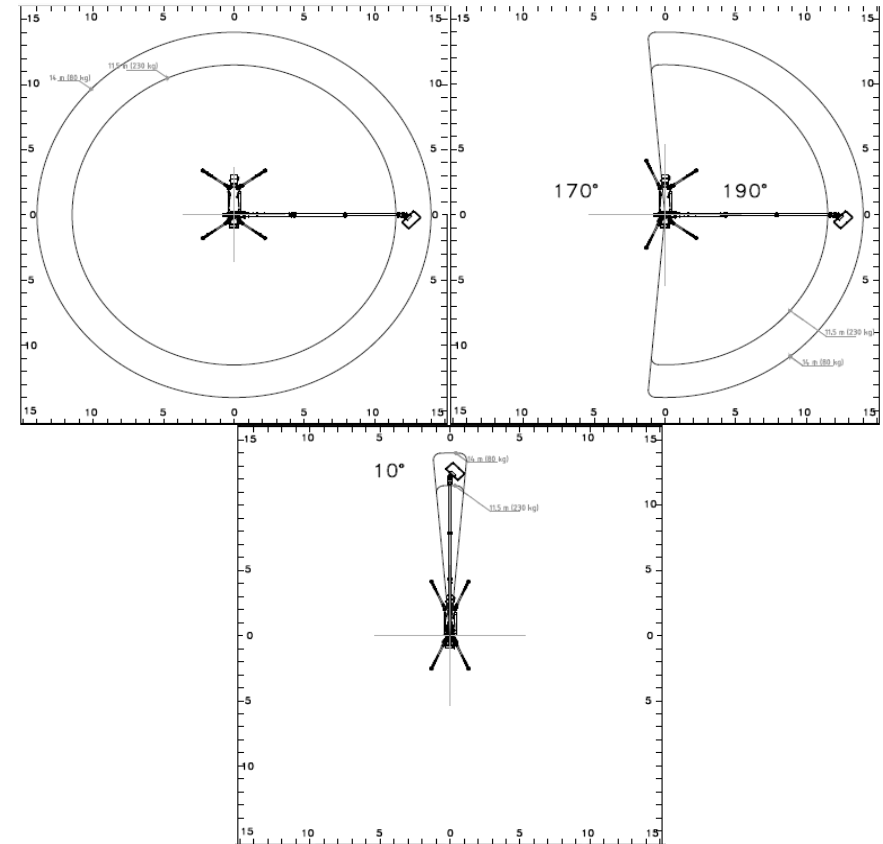
Afbeelding 2b: arbeidsområder.
